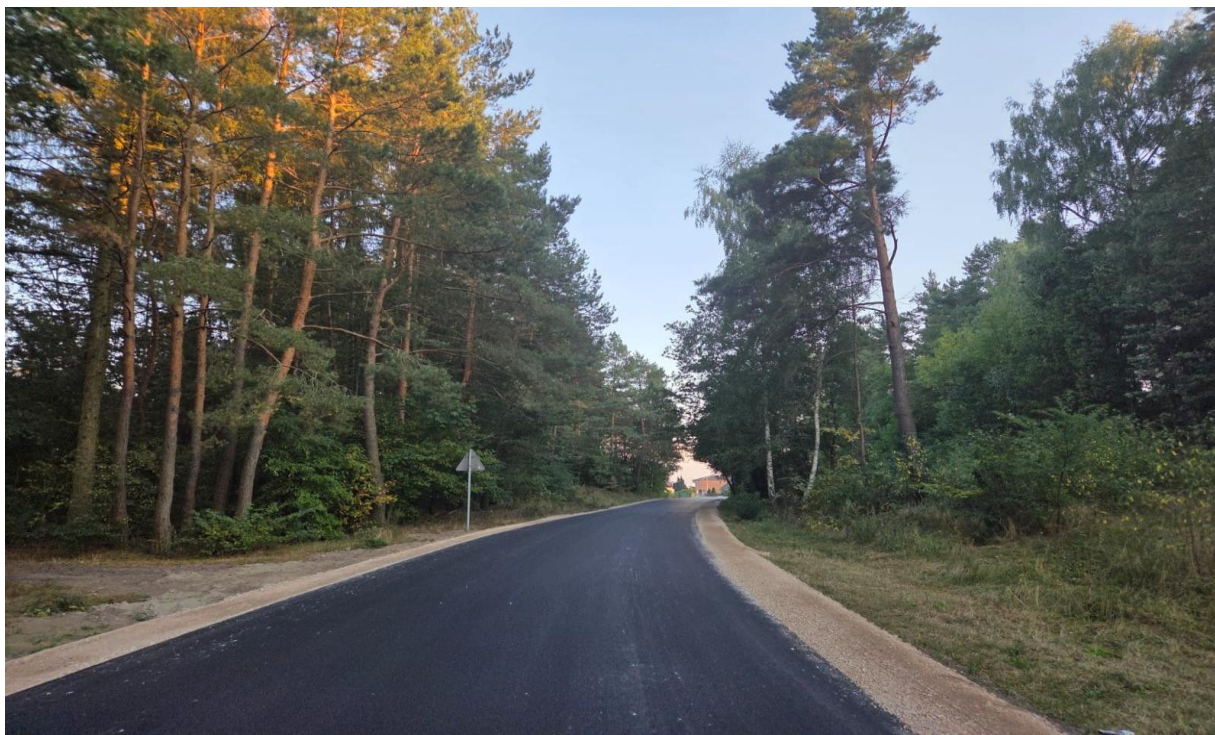
Zdjęcie 5.2.5. Przebudowa drogi gminnej nr DG110208E w Kalinkach
