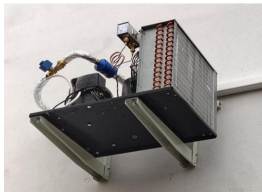
Zdjęcie 5.4.8. i 5.4.9 Agregat chłodniczy do chłodni w budynku strażnicy OSP w Kraszewicach
